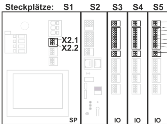
a) RWA-Zentrale mit drei Input/Output-Modulen
