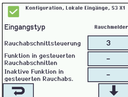
Konfiguration der lokalen Eingang S3 auf X1
