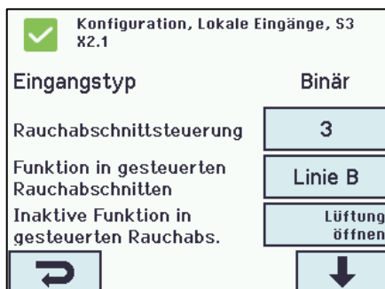
Konfiguration die lokalen Eingänge X2 und X5
