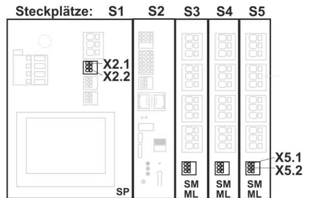
b) RWA-Zentrale mit drei Motormodulen
